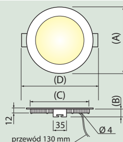
Wymiary oprawy
